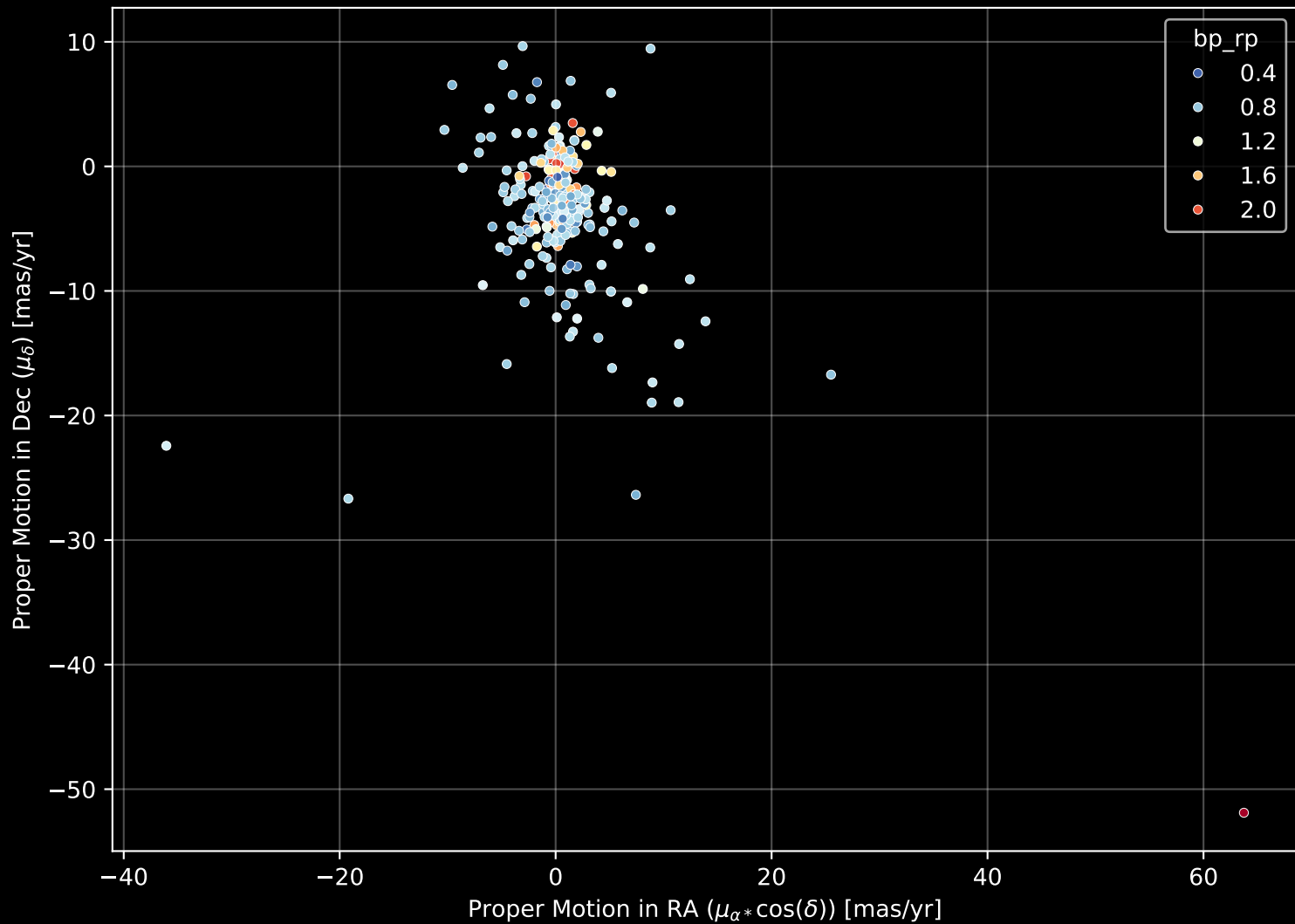
GALAH DR4 Field: [9469] Proper Motion Diagram (n= 283)
