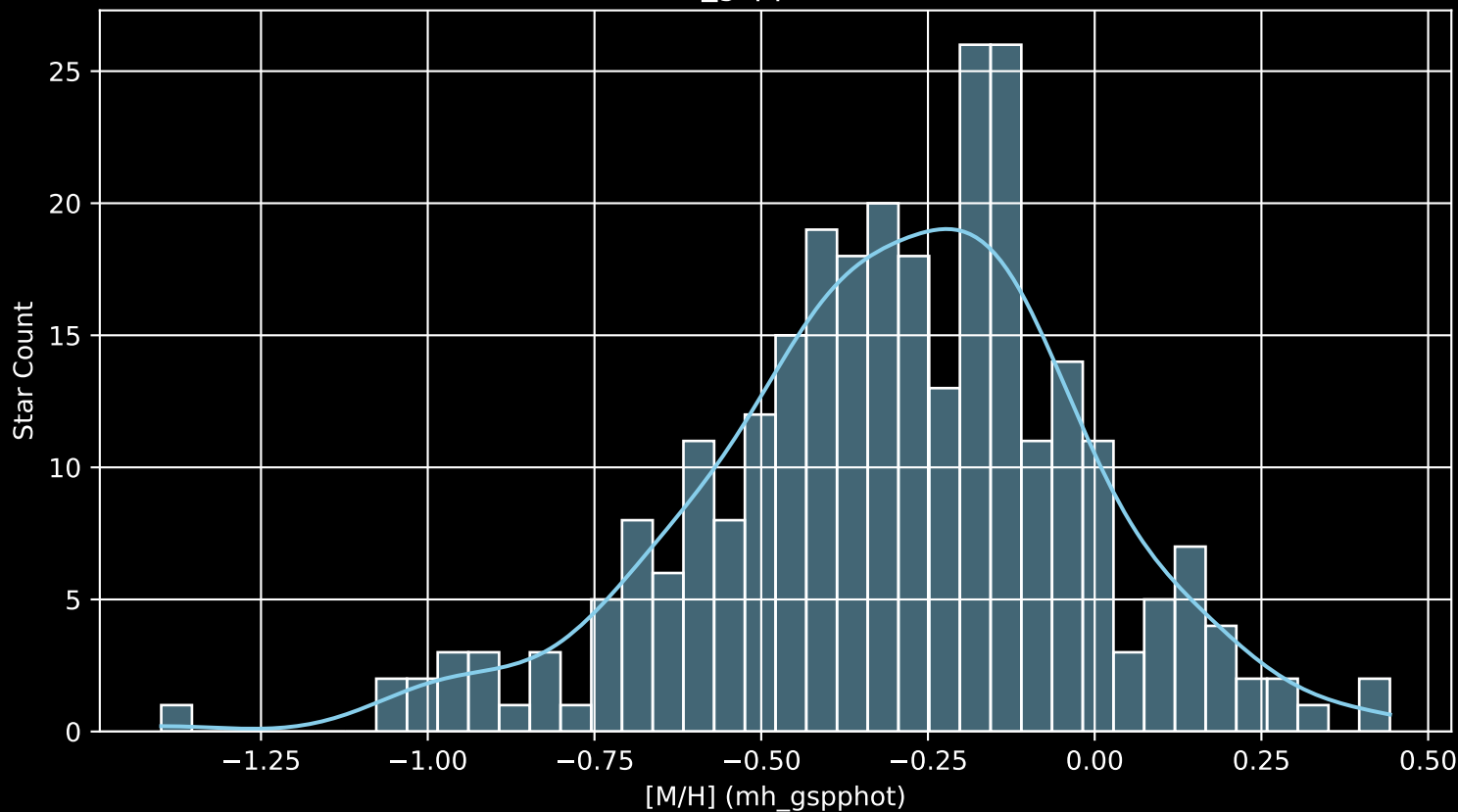
GALAH DR4 Field: [9469] [M/H] (mh_gspphot) (n= 283)
