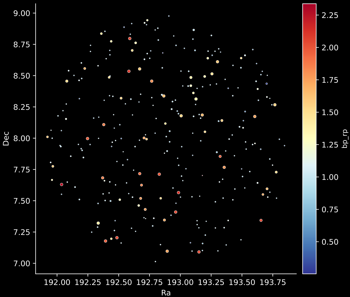
GALAH DR4 Field: [9469] Stars: 283
