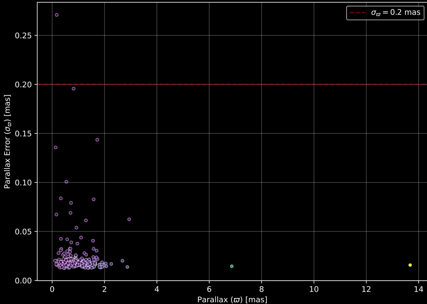
GALAH DR4 Field: [9469] Parallax Quality (n= 283)
