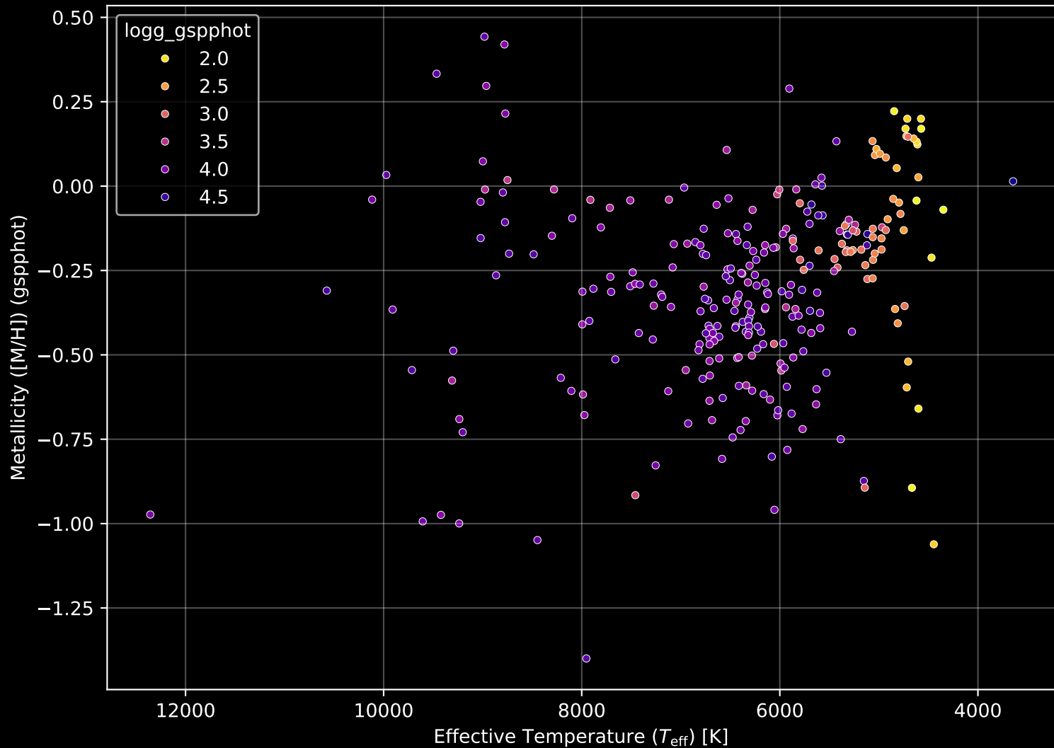
GALAH DR4 Field: [9469] Stellar Population Parameters (n= 283)
